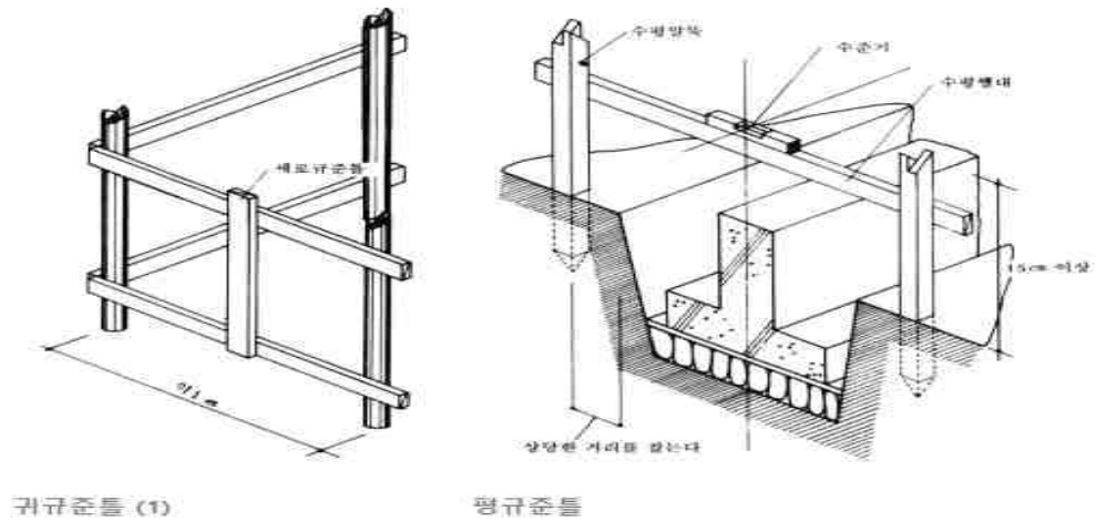
[그림 1] 평·귀기준틀 상세도
